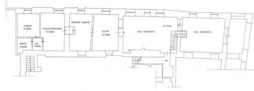
PIANTA PIANO TERRENO
