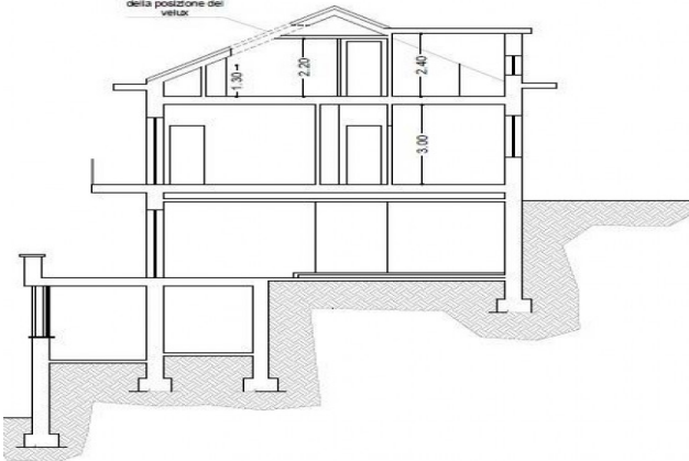
SEZIONE A - A' scala 1/100
