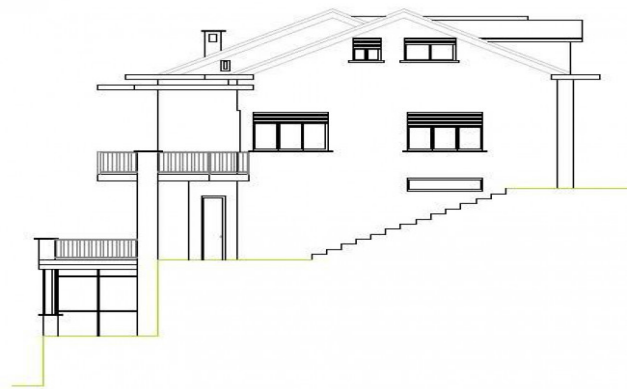
PROSPETTO SUD
