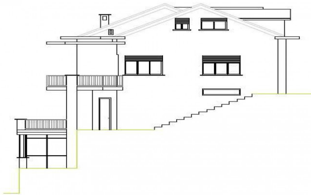
PROSPETTO SUD
