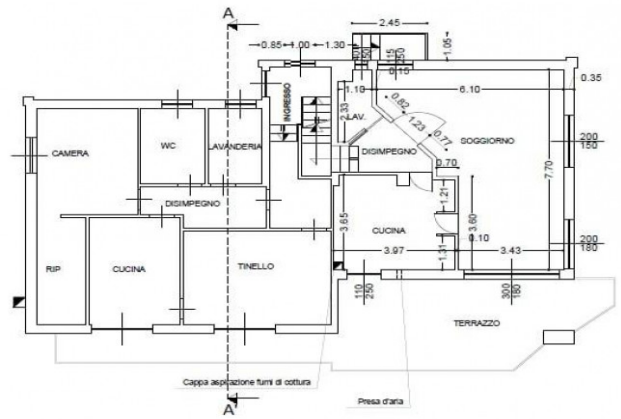
PIANTA PIANO RIALZATO scala 1/100
