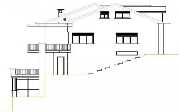
PROSPETTO SUD
