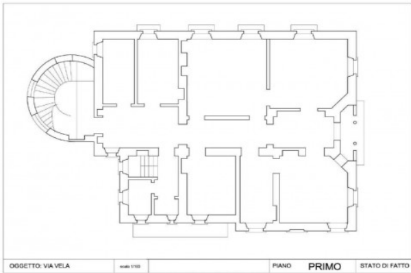
OGGETTO: VIA VELA scala 1:100 PIANO PRIMO STATO DI FATTO
