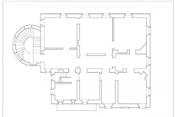
OGGETTO: VIA VELA scala 1:100 PIANO SECONDO STATO DI FATTO
