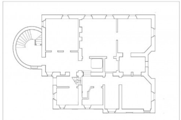
OGGETTO: VIA VELA scala 1:100 PIANO INTERRATO STATO DI FATTO
